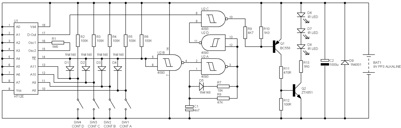
燈光控制 - 遙控發射器
